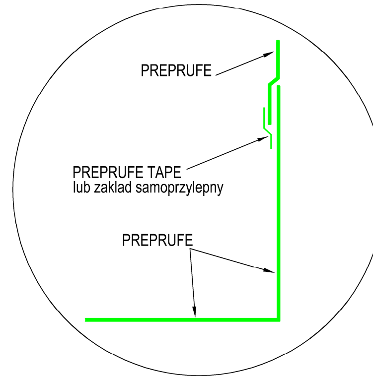
ALTERNATYWNA APLIKACJA PREPRUFE W NAROŻU
