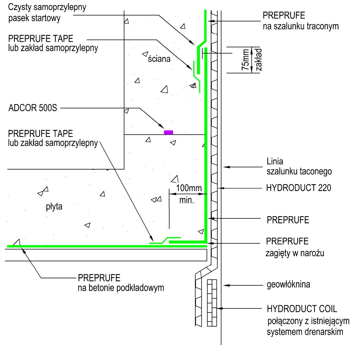
DETAL NAROŻNIKA Z DRENAŻEM PRZEKRÓJ
